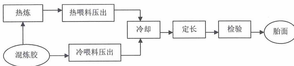
图3-3 压延压出工段工艺流程图
