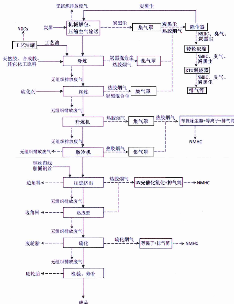
图3-1 本项目生产工艺及产污节点图
