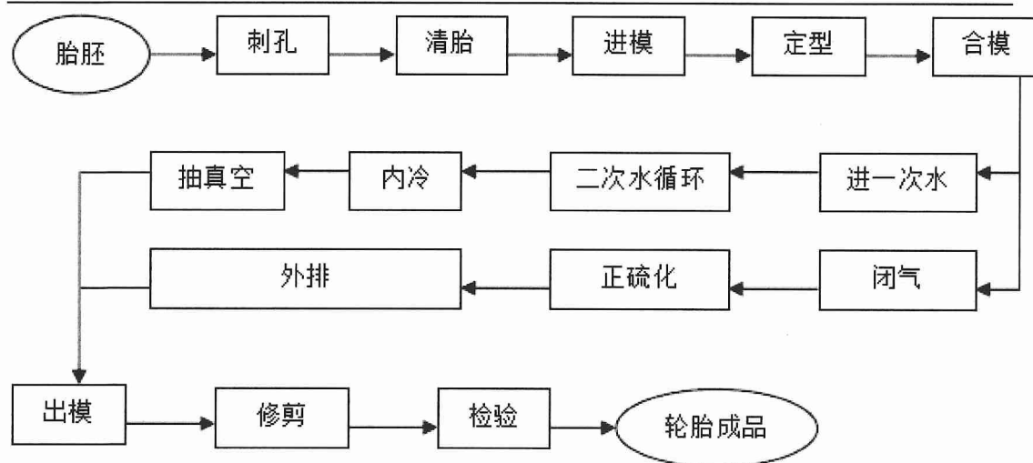
图 3-5 硫化工段工艺流程图
