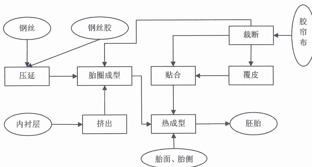
图3-4 成型工段工艺流程图
