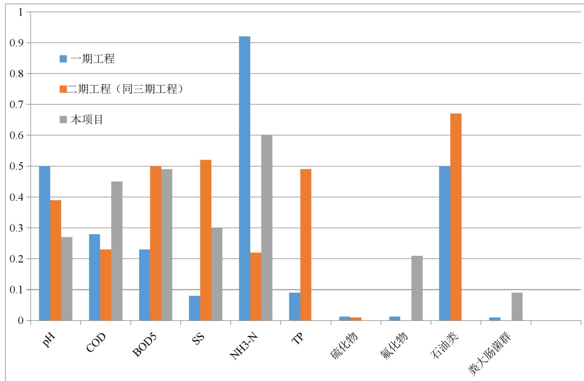
图 3.2-2 W3 监测断面各工程环评时期监测因子标准指数变化趋势图
