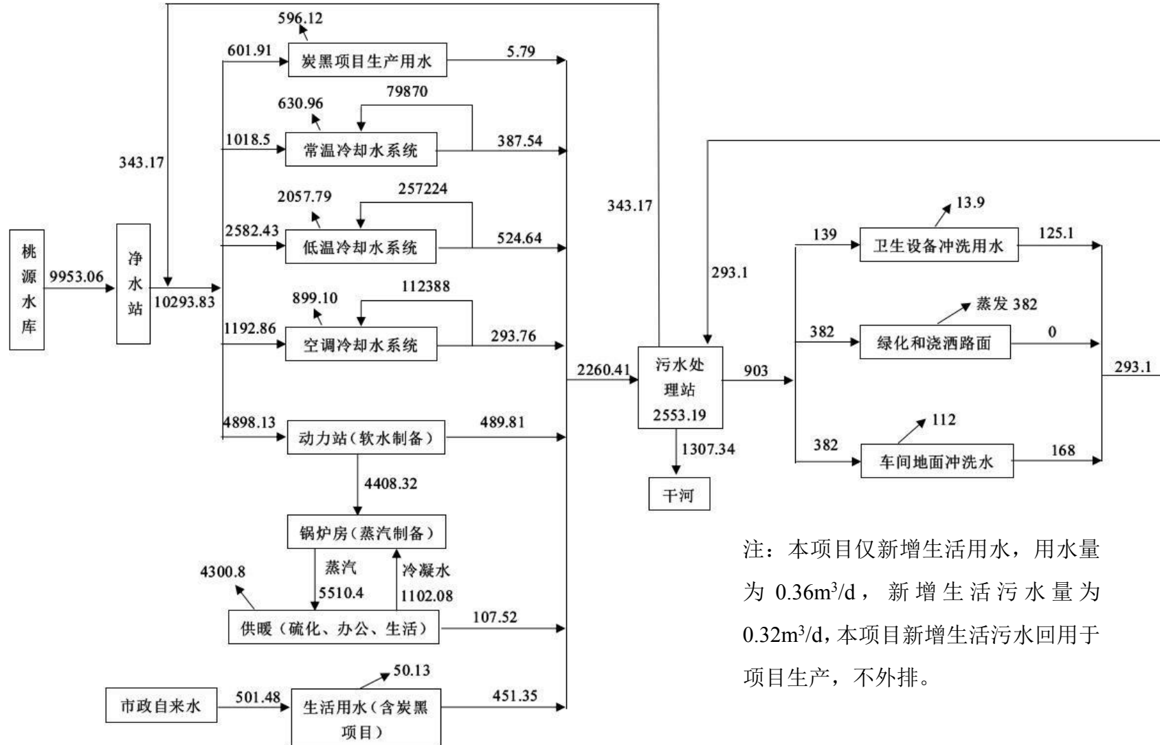
图 2.1-4 本项目建成后全厂水平衡图 单位：m³/d
