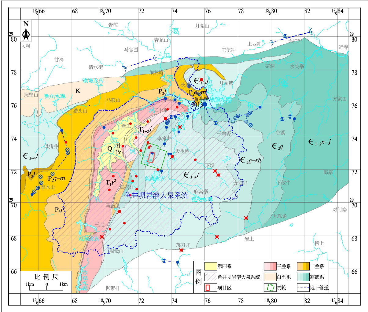
图 4.2-1 区域地层平面图
