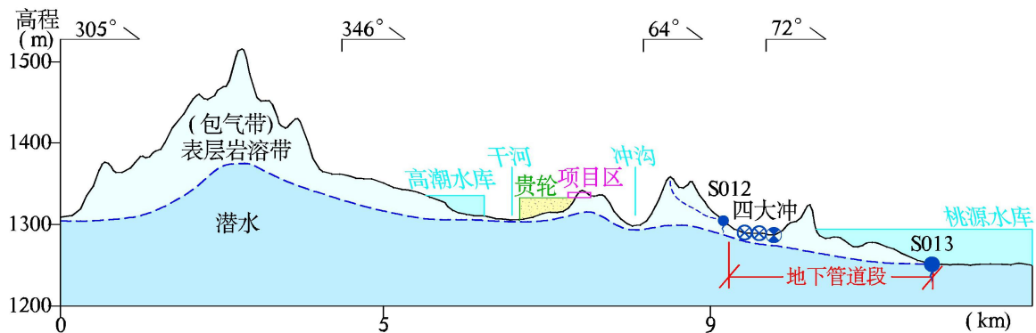
图 4.2-8 项目与 S103 鱼井坝岩溶大泉的剖面关系示意图
