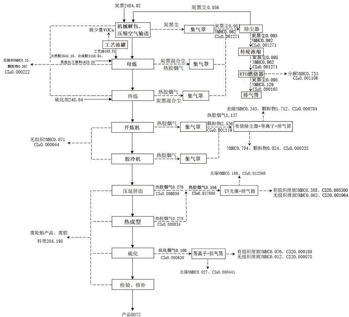
图 2.1-2 本项目主要物料平衡图 单位 t/a
