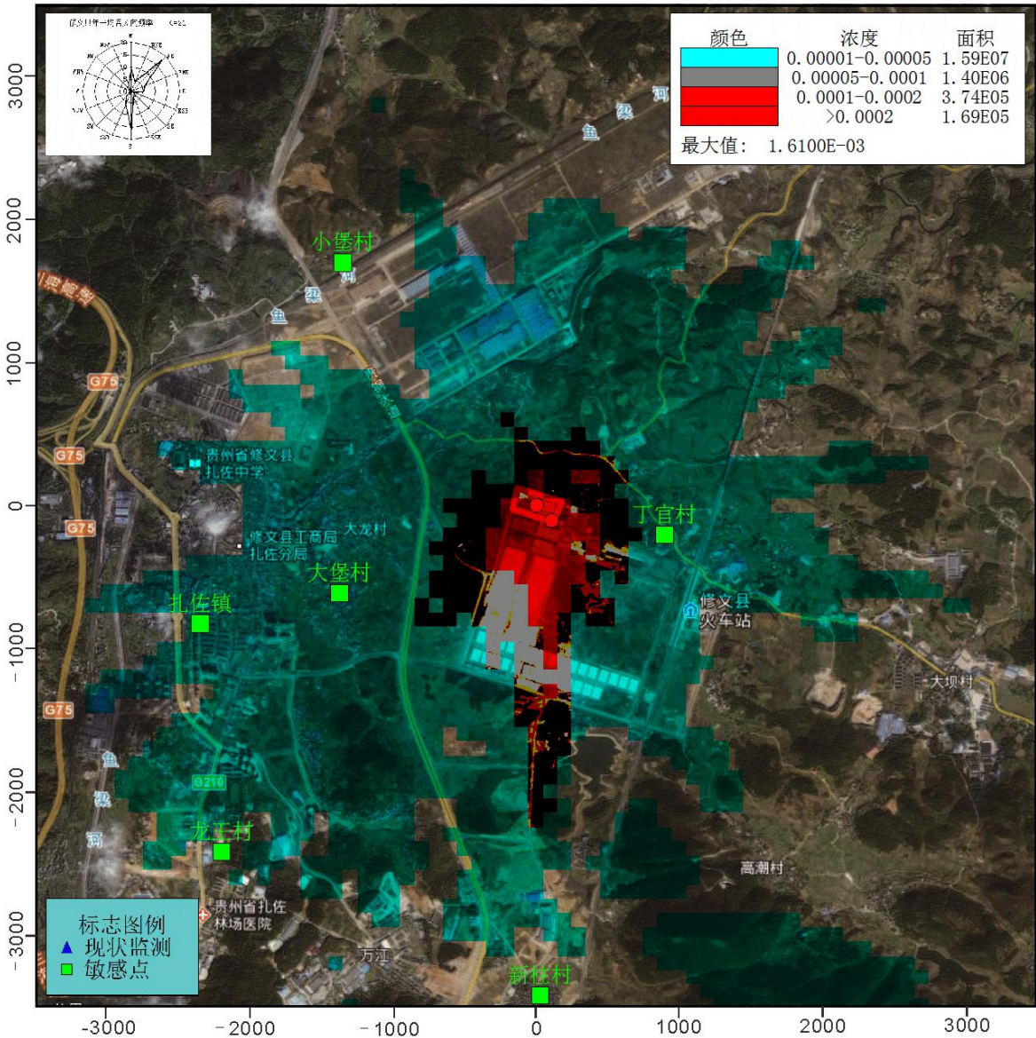
图 4.3-17 网格点 NMHC 日均浓度分布图
