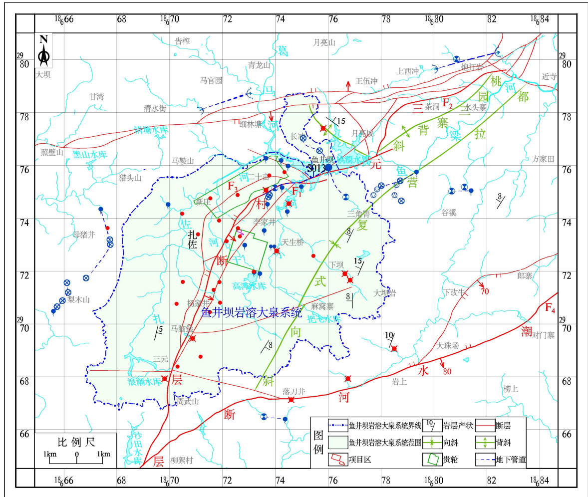
图 4.2-2 区域地质构造纲要图
