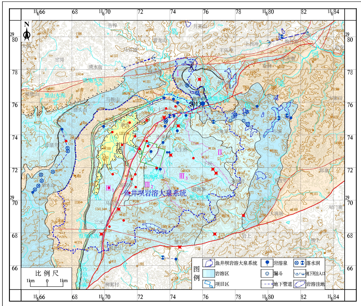
图 4.2-3 区域岩溶发育平面分布图
