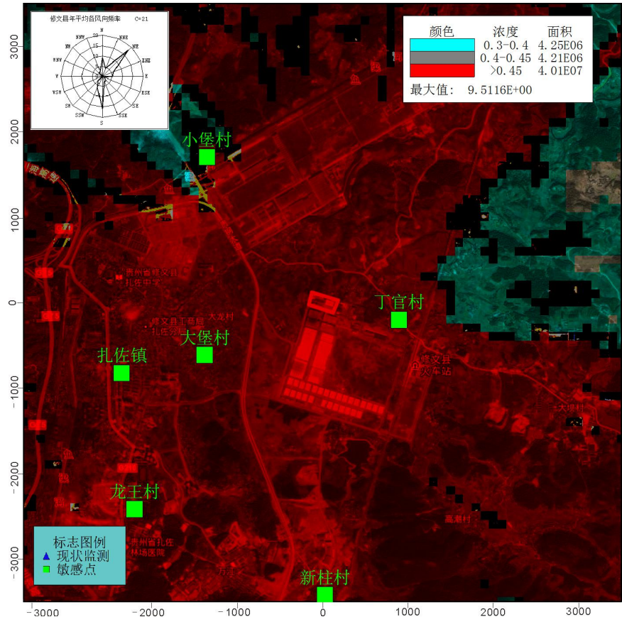
图 4.3-37 事故情况 3 下网格点 \text{PM}_{10} 小时平均质量浓度分布图
