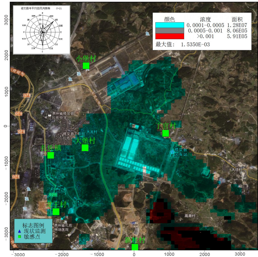
图 4.3-19 网格点 NH 3 小时浓度分布图
