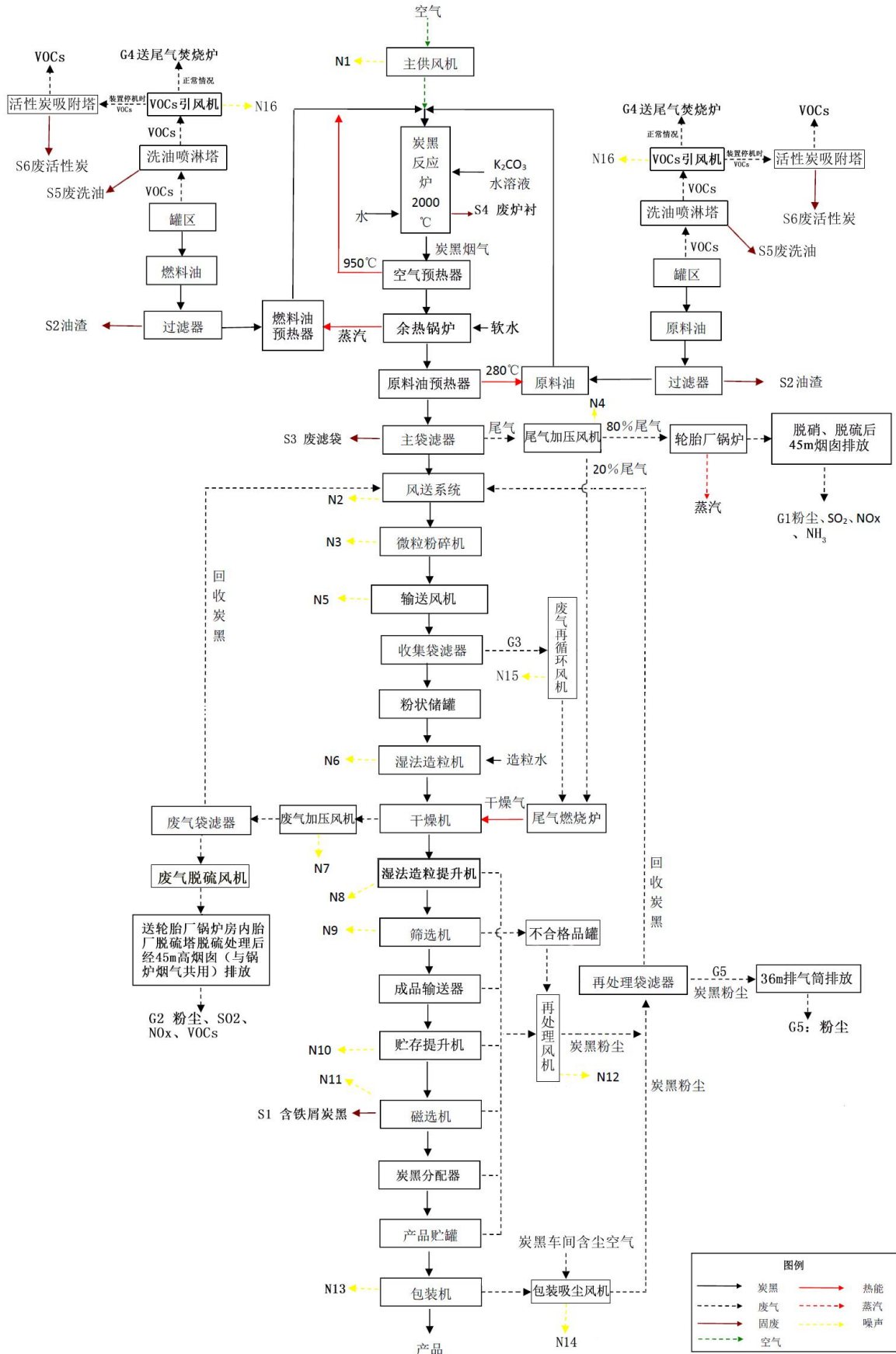
图 2.3-2 本项目工艺流程及产污节点图
