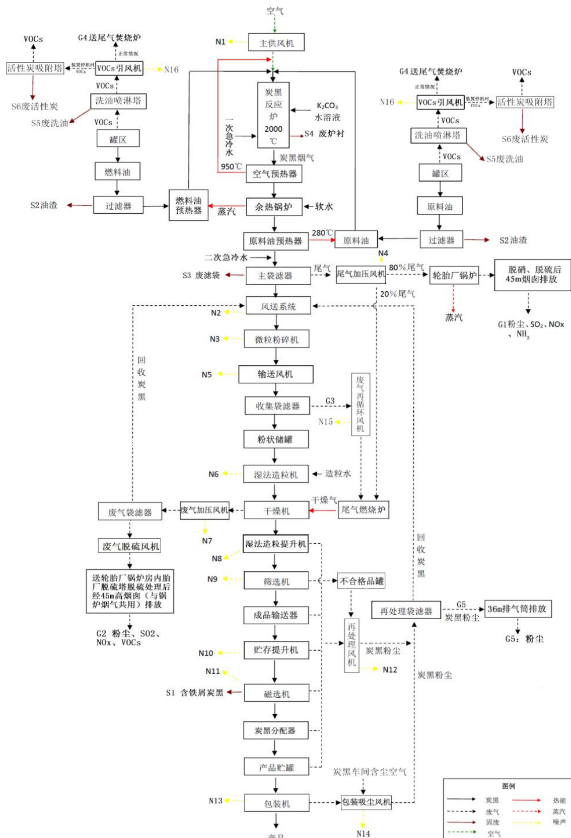
图 6.1-1 生产工艺流程图
