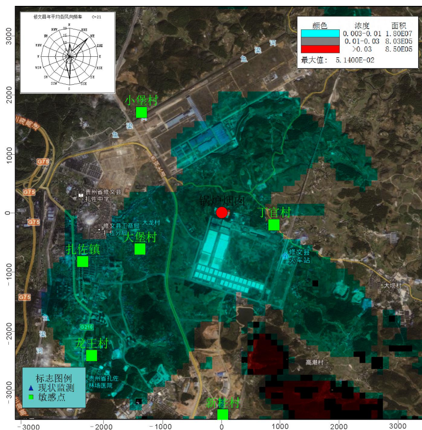
图 4.3-6 网格点 SO 2 小时浓度分布图
